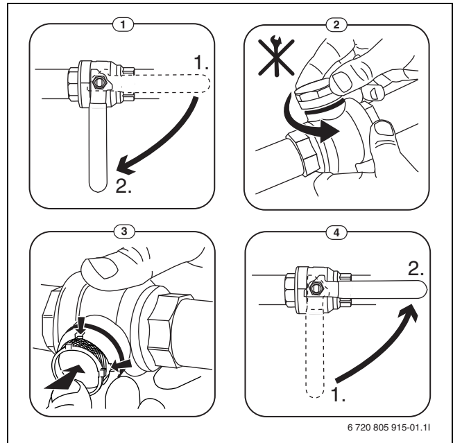
Afb. 7 Filterreiniging
